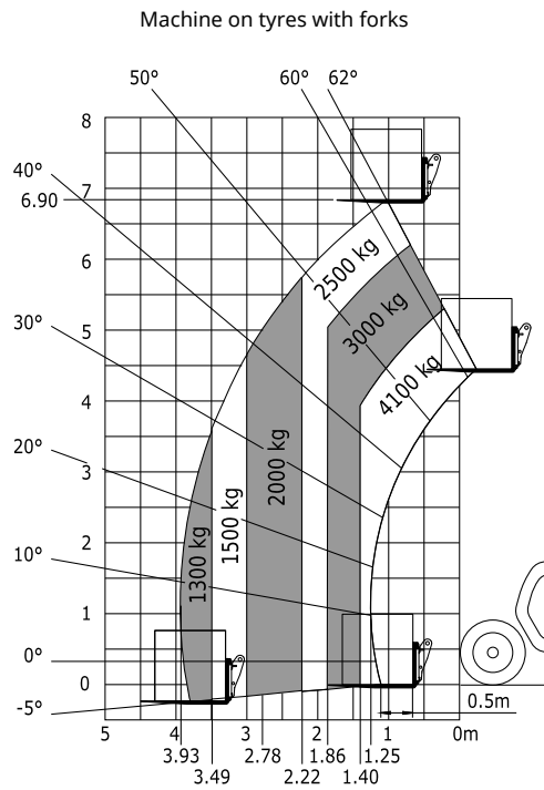
Rough terrain load chart (EN 1459 B)
